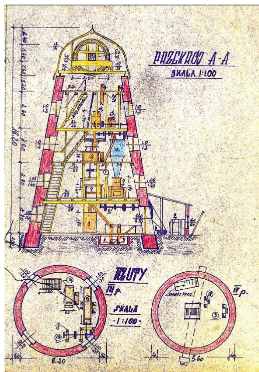
Rys. 123. Przekrój wiatraka w Zagoździe, 1960r., ze zb. M.Krasnowskiego
