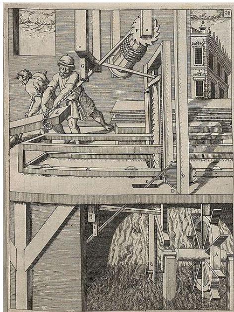
Rys. 2. Folusz wodny oraz młyn tartaczny wg grafik Georga Andreasa Boecklera z 1661r.
